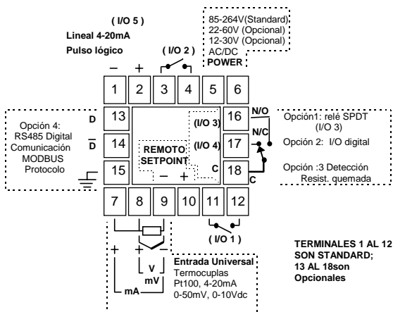
Figura 2 - Conexiones del panel trasero.
