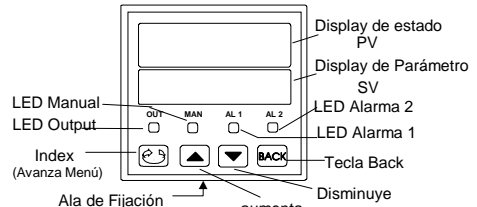
Figura 1 - Identificación de las partes del panel frontal
