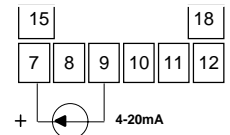
Figura 6 - conexión de corriente
