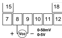
Figura 4 - conexión de tensión
