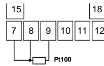
Figura 5 - conexión de Pt100 a 3 hilos
