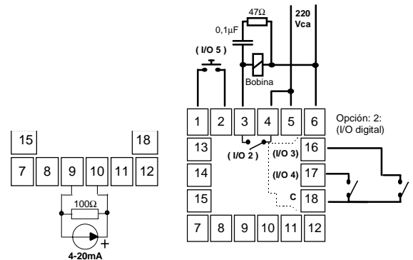
Figura 7 - conexión para SP remoto
